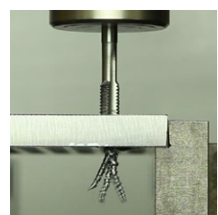
POでの切りくず排出状況
