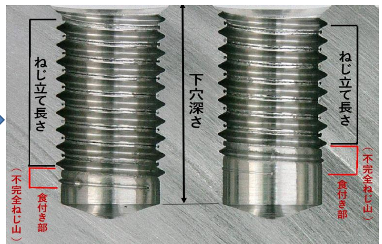
加工後のめねじ断面図
