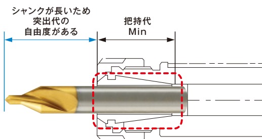
片刃タイプセンタ穴ドリルの場合
