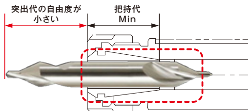
両刃タイプセンタ穴ドリルの場合
