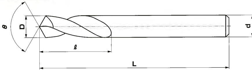
先端角(θ): NC-SD-V 90° NC-SD 125°
